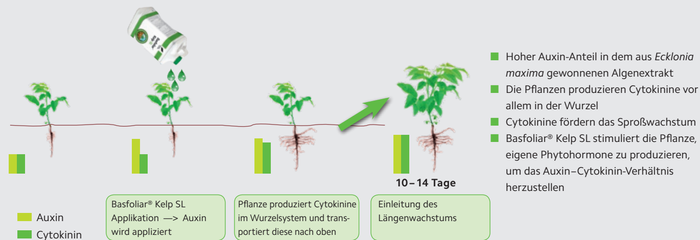
Abb. 12: Effekte der in Algen enthaltenen Auxine und Cytokinine
