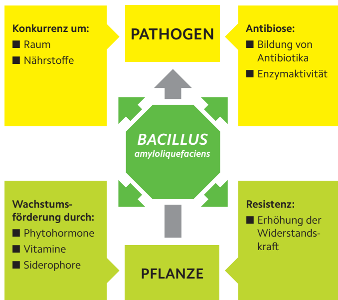
Wirkmechanismen von nützlichen Rhizosphärenbakterien (Grafik Dr. Lord)
