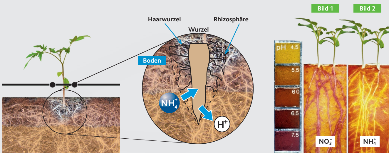
Abb. 3: Wirkung unterschiedlicher N-Ernährung in der Rhizosphäre
