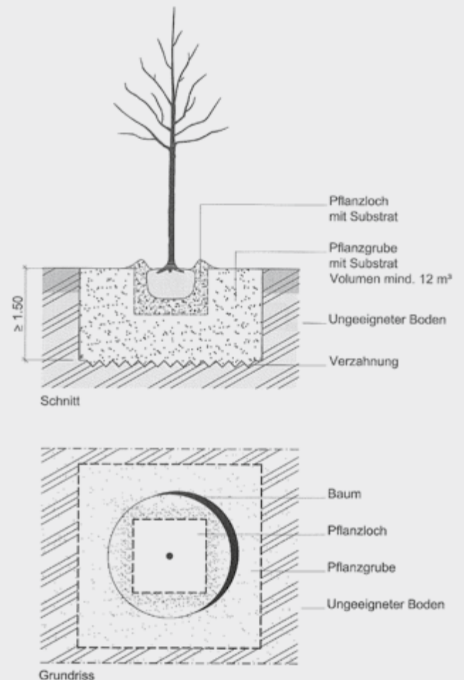
Abb. 38: 2 FLL Pflanzgruben-Skizzen
